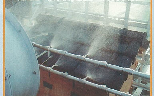
積雪地での棟上部取付型製品との換気試験
